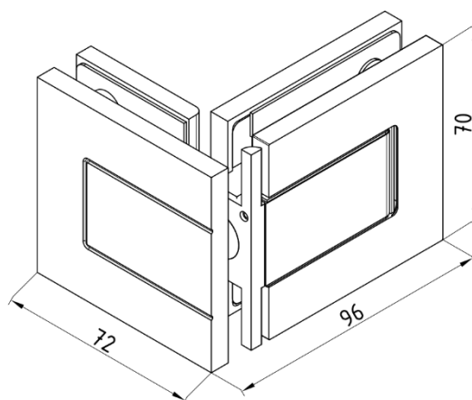
Variante mit Dichtung
