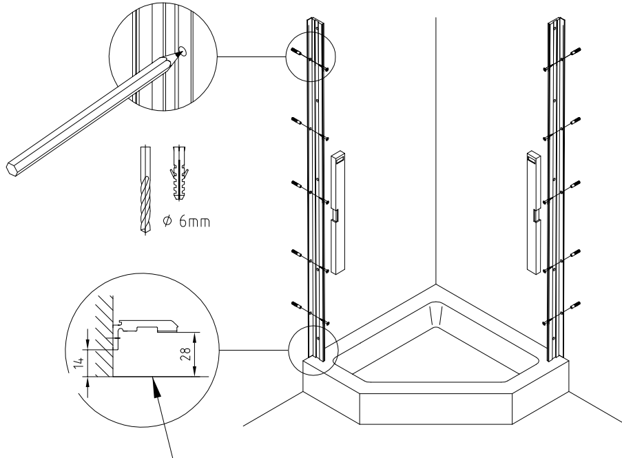
Duschwannen Außenkante Shower tub outer edge
