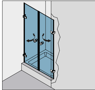
Typ(e) 105 Nischenkabine, 2 Pendeltüren
