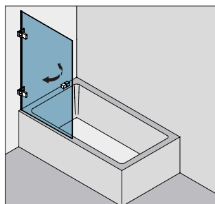
Typ(e) 170 Eckkabine, 1 Pendeltür auf Badewanne 90°
